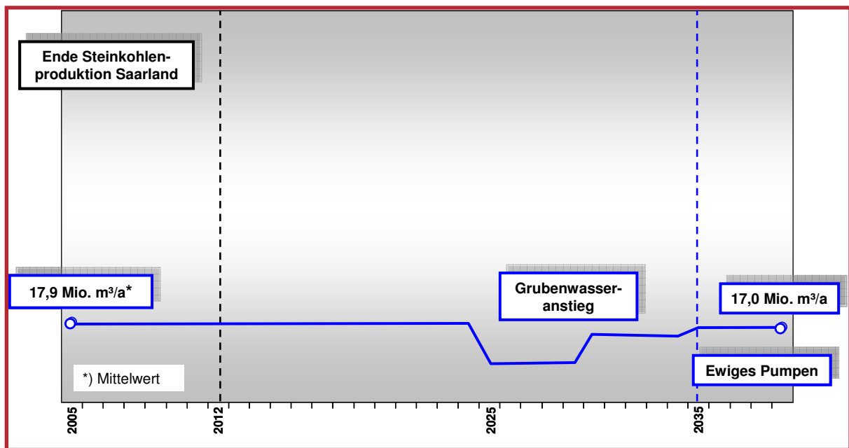
Abbildung 1: Grubenwassermengenentwicklung Saarland
